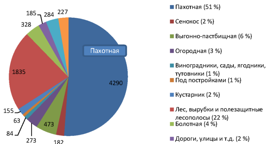
Рис. 2. Состав земель по основным видам угодий по Краснодарскому краю на 1 ноября 1945 г. (тыс. га) [8, л. 84]
