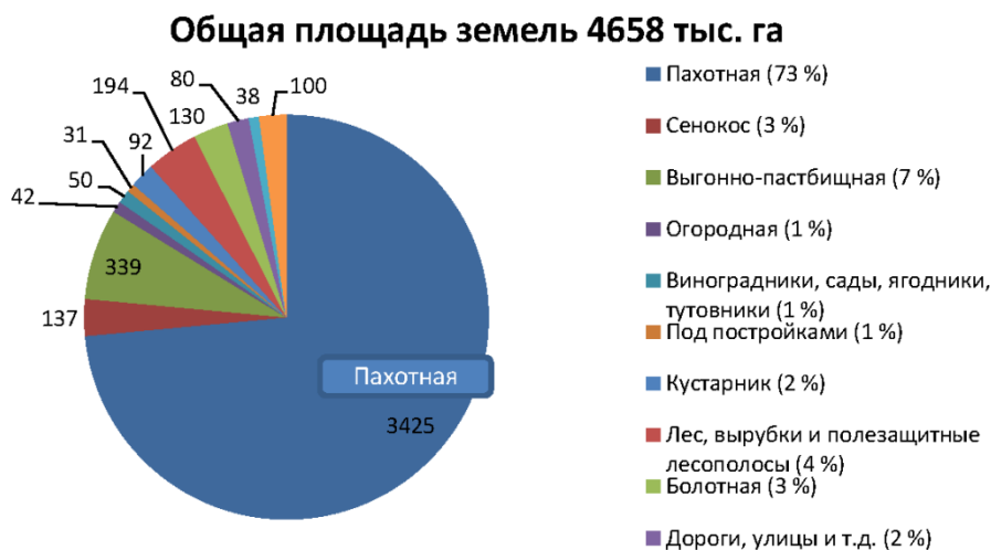
Рис. 3. Состав обобщественных земель колхозов по основным видам угодий Краснодарского края на 1 ноября 1945 г. (тыс. га) [8, л. 85]
